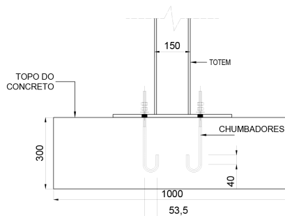
BASE DO TOTEM SEM ESCALA
