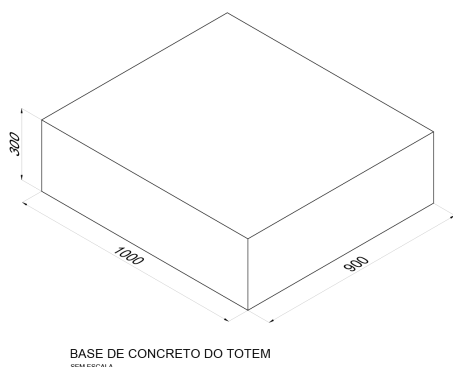
BASE DE CONCRETO DO TOTEM SEM ESCALA
