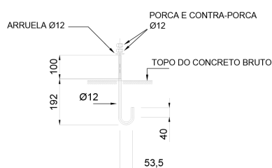
CHUMBADOR Ø12 L=401 mm
